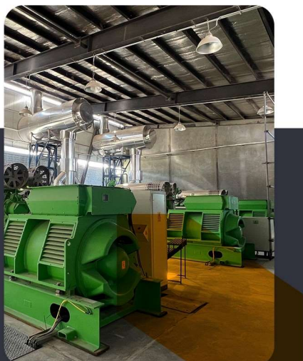
۳ دستگاه مولد JENBACHER مدل 620 توان ۳۴۵۰ کیلو وات
