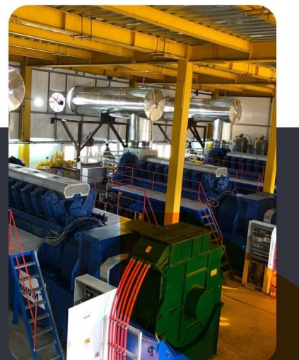
۳ دستگاه مولد MWM مدل TCG2032V16 توان ۴۳۰۰ کیلو وات
