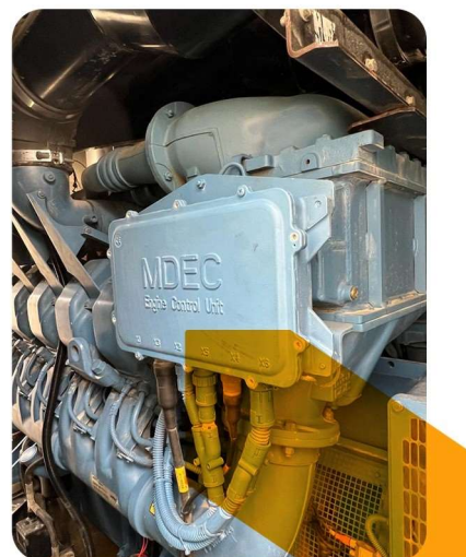
۲ دستگاه مولد دیزلی MTU مدل 12V4000 توان ۱۵۰۰ کیلووات
