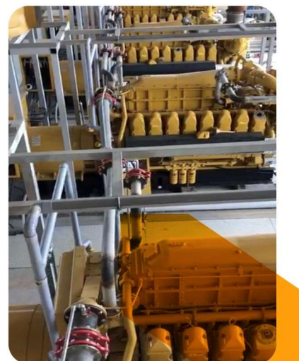
۵ دستگاه مولد CATERPILLAR مدل G3516C توان ۱۶۰۰ کیلو وات
