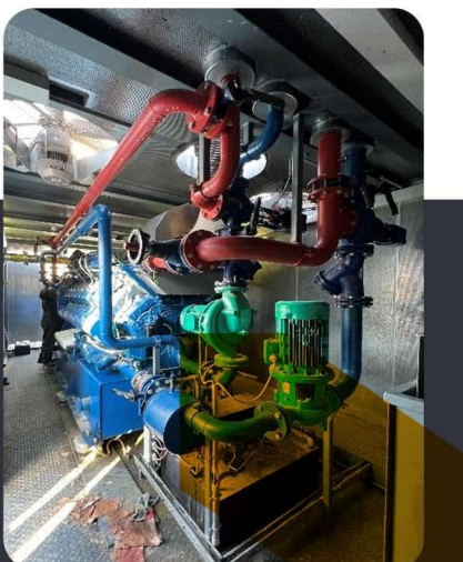
۱ دستگاه مولد MWM مدل TCG2020V16 توان ۱۵۶۰ کیلو وات
